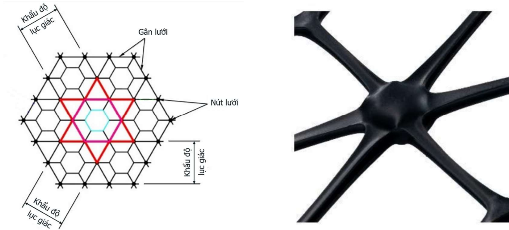
Hình 1. Hình dạng Lưới địa kỹ thuật ổn định nền Tensor HX165
